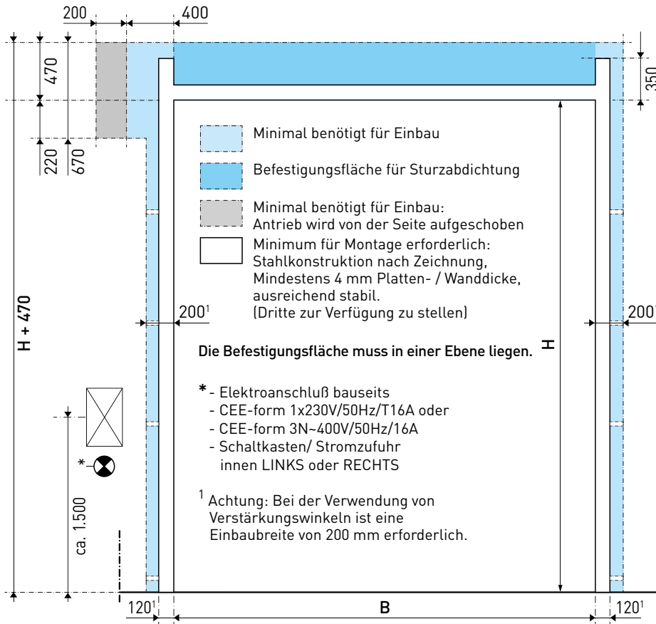
[ Antriebsseite ]
