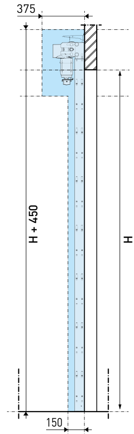
[ Leiterquerschnitt ]
