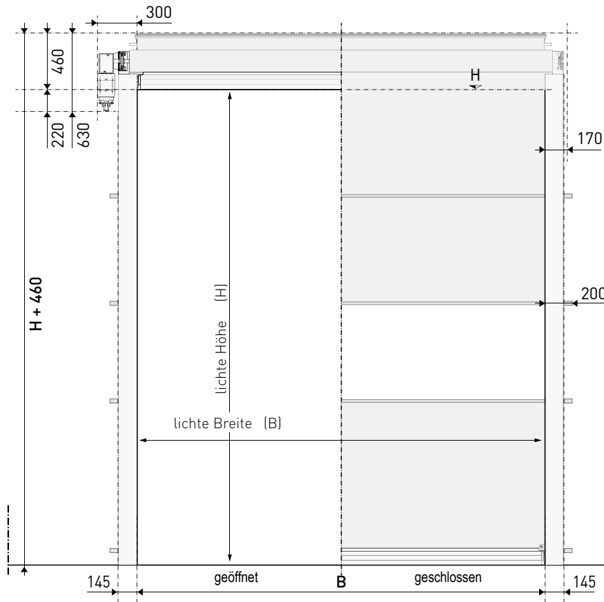
[ Antriebsseite ]
